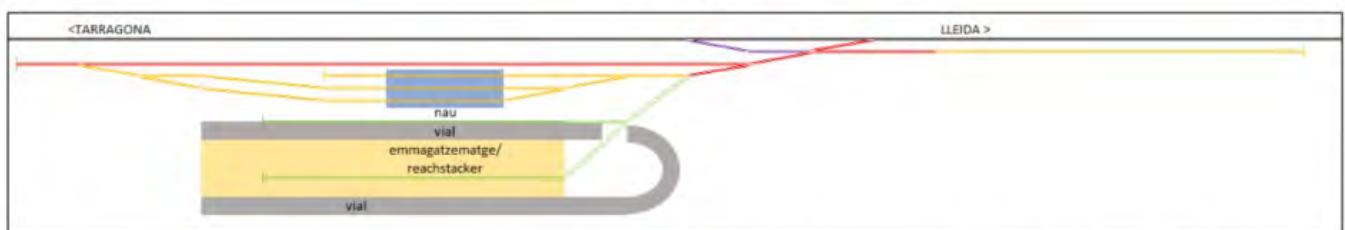
Esquema de vies de l'escenari 1A (Llegenda: negre: RFIG; vermell: vies existents; lila: nou enllaç; groc: R/E i cua de maniobres; verd: C/D)
