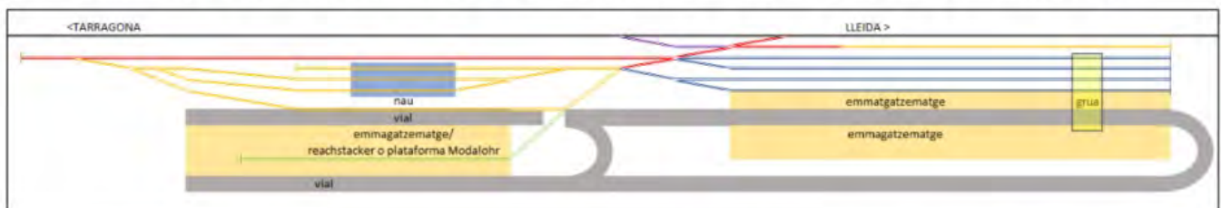
Esquema de vies de l'escenari 1A+3 (Llegenda: negre: RFIG; vermell: vies existents; lila: nou enllaç; groc: R/E i cua de maniobres; verd: C/D, blau: C/D fase ampliació)
